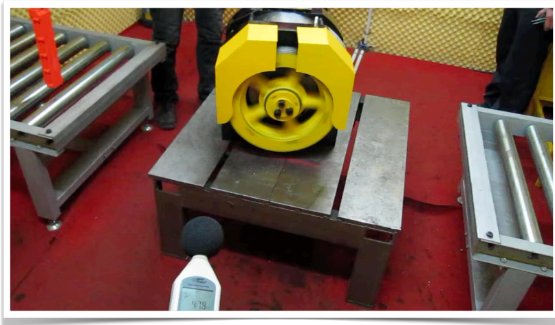
최첨단 저소음 권상기 적용
